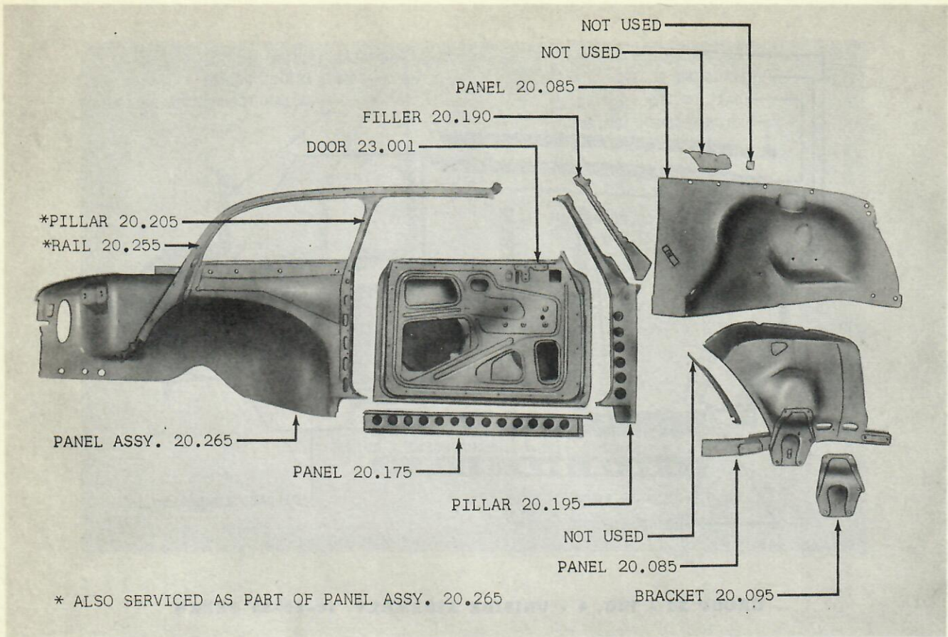
GROUP 20 - FIG. 6 - BODY SIDE PANELS 01 SEDAN
